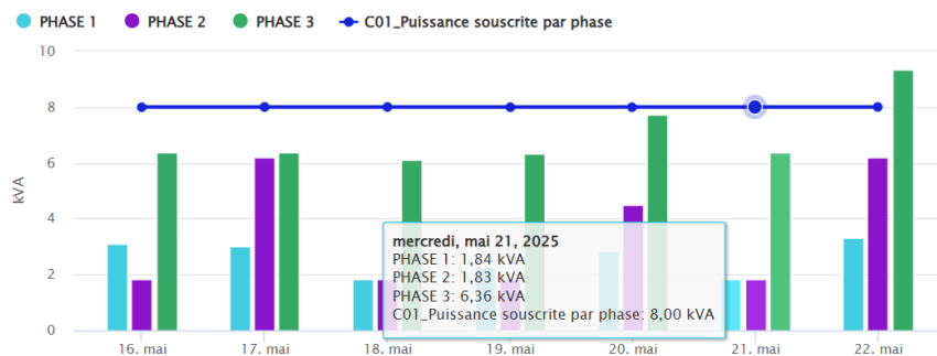
PMax atteinte journalière vs Puissance souscrite par phase (kVA)
